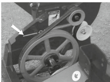
Настраивающий болт
