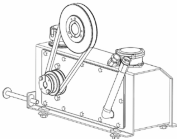
Рис. 39. Гидравлический приводной блок для моделей: ВХ42R & ВХ62R.
