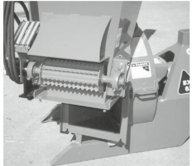
Загрузочный бункер
