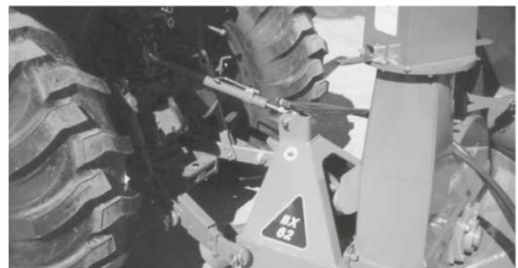
Рис. 19. Верхняя тяга.
