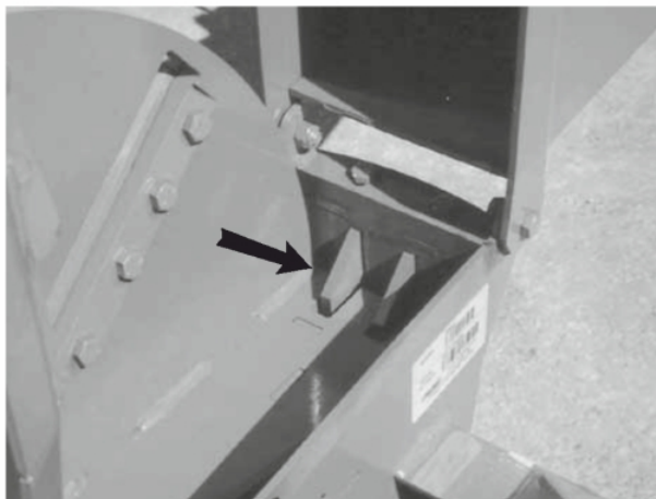
Расположение дробилки внутри роторного отделения
